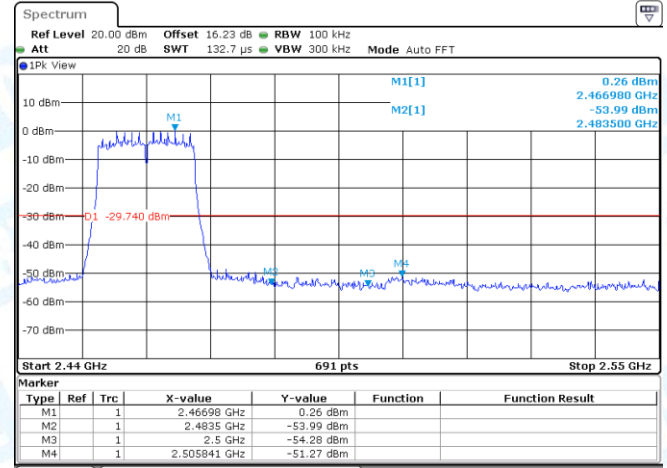
11G-CDD-Ant2-2462-PASS
