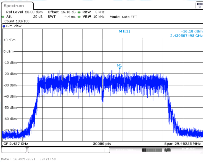
11AX20MIMO-Ant1-2437-PASS
