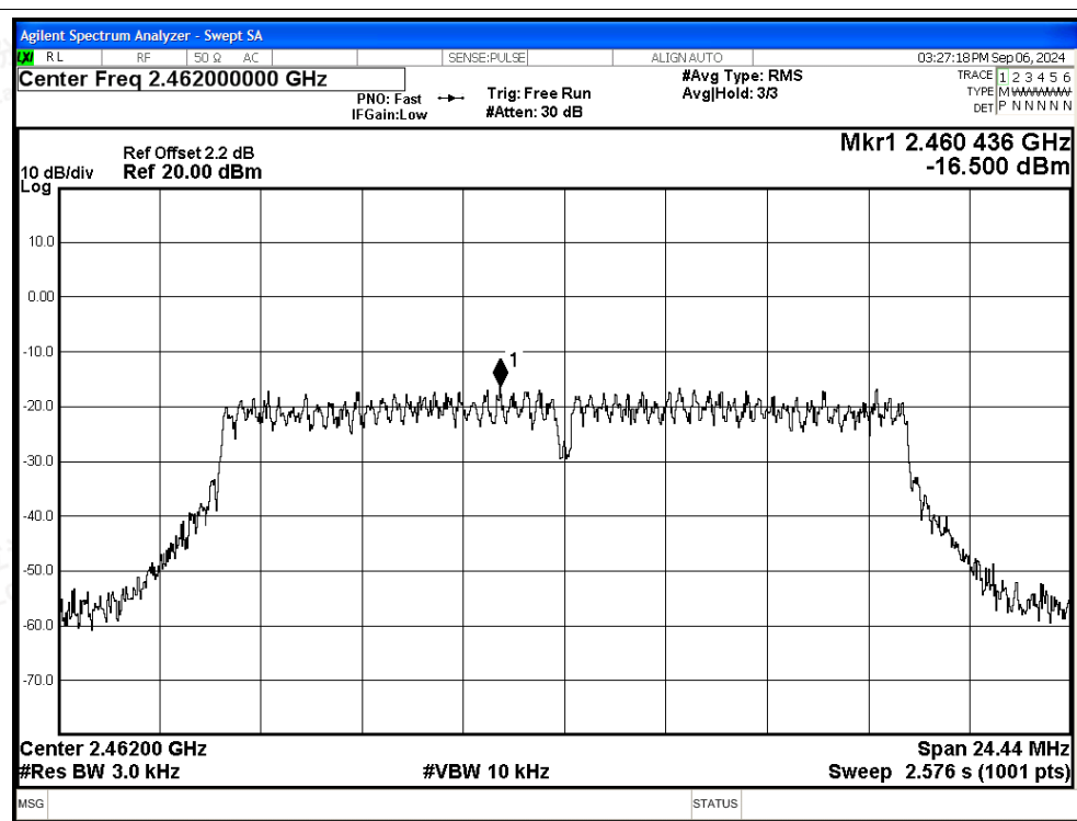
PSD NVNT g 2462MHz Ant
