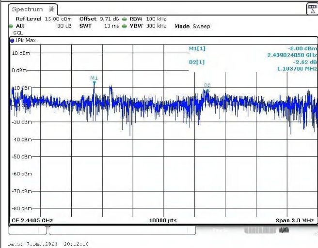
8DPSK
