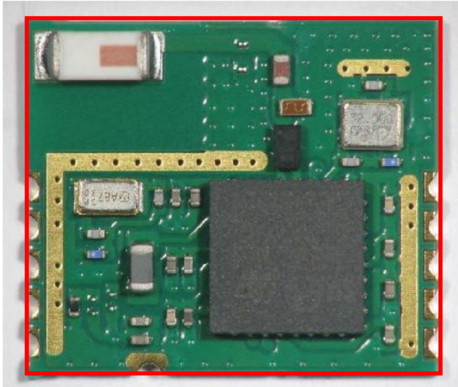
BLE Module without the shield plate
