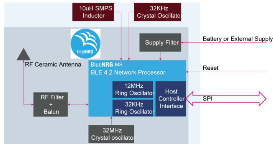
BLE Module (detail)
