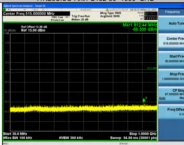
11N20SISO-Ant1-2462-1000~26500--2.12
