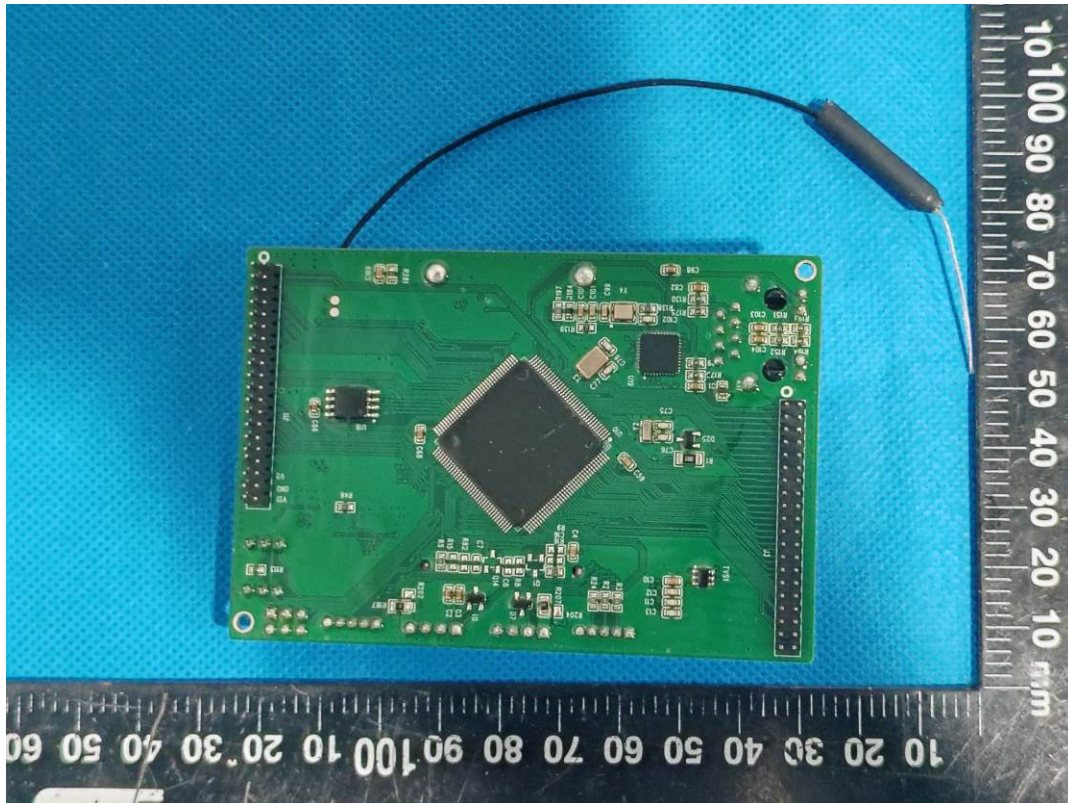
PLC Module
