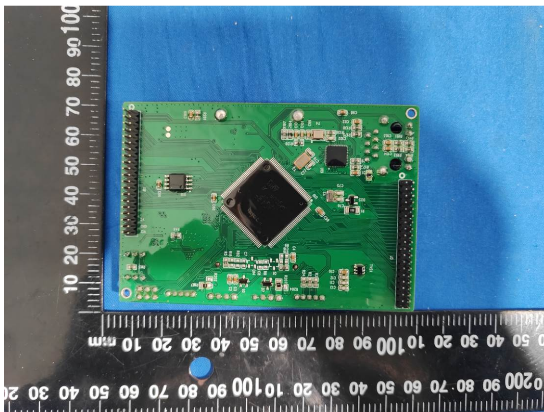
WWAN Module
