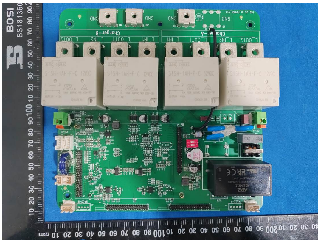
PLC Module
