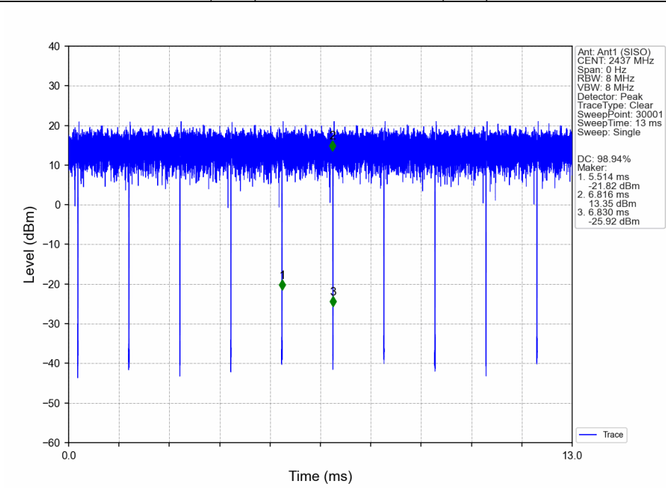
802.11n(HT20)_MCH_2437MHz_Ant1 (SISO)_NTNV
