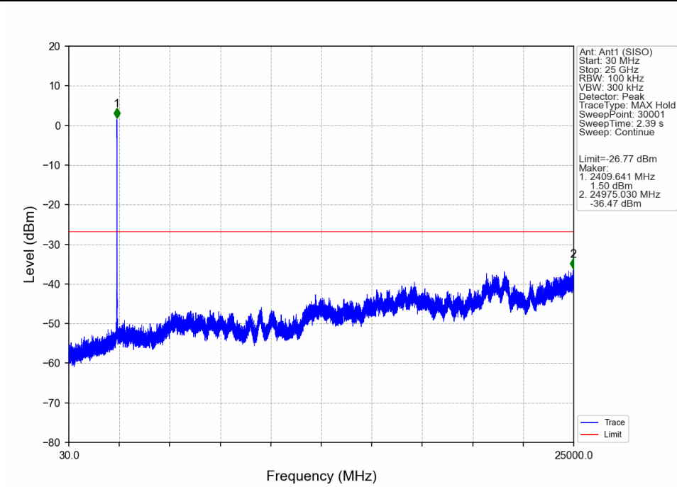
802.11g_LCH_2412MHz_Ant1 (SISO)_NTNV
