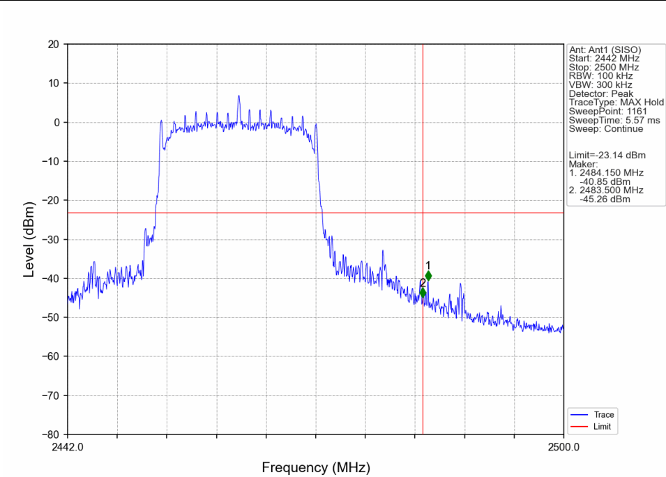
802.11n(HT20)_HCH_2462MHz_Ant1 (SISO)_NTNV
