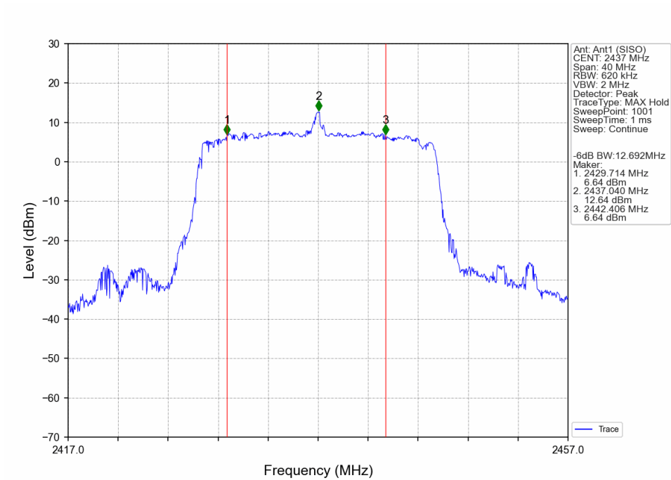
802.11n(HT20)_MCH_2437MHz_Ant1 (SISO)_NTNV
