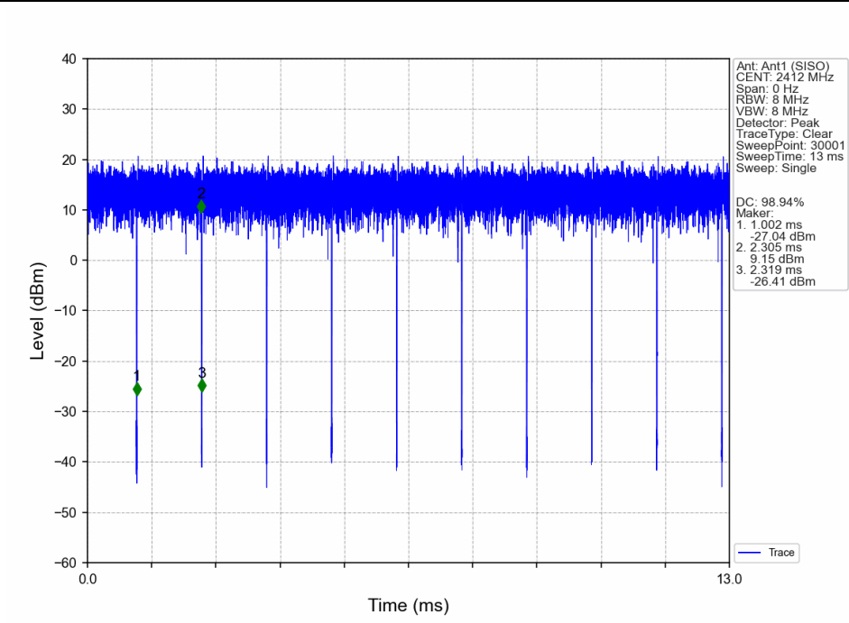
802.11n(HT20)_LCH_2412MHz_Ant1 (SISO)_NTNV
