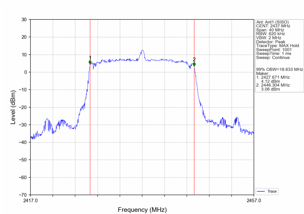
802.11n(HT20)_MCH_2437MHz_Ant1 (SISO)_NTNV
