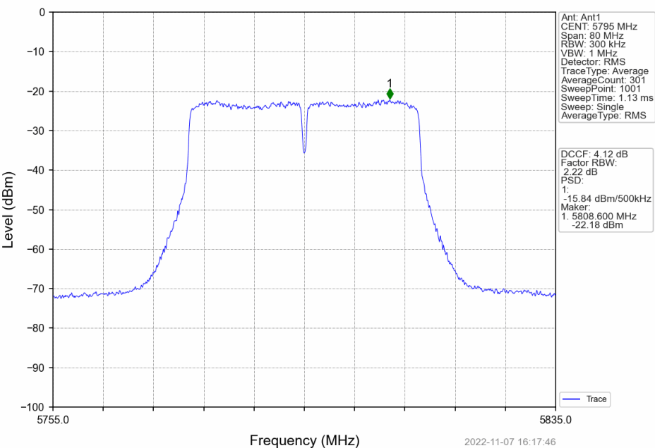
802.11n(HT40)_HCH_5795MHz_Ant1 NTN
