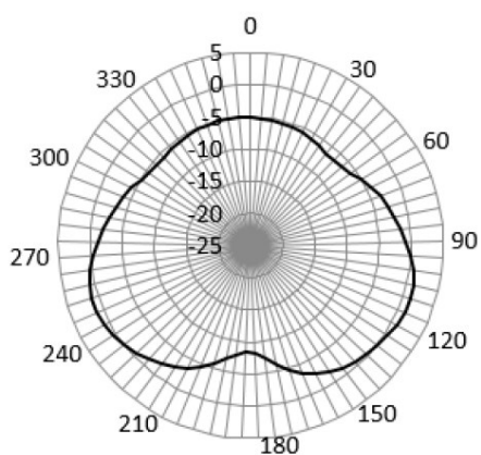
YZ-912MHz
