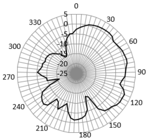
XZ-2450MHz
