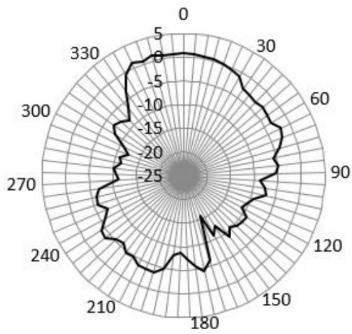
XZ-5450MHz
