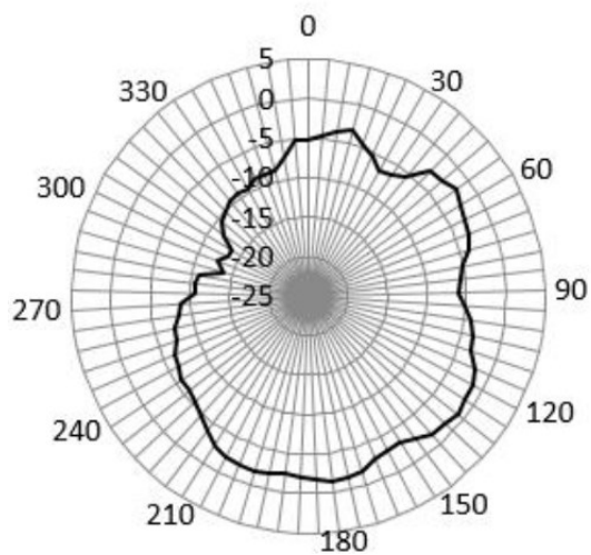
XY-5450MHz
