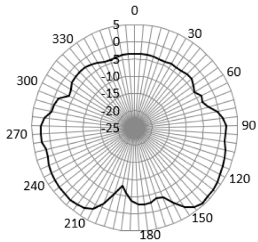
YZ-2450MHz
