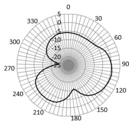
XZ-912MHz
