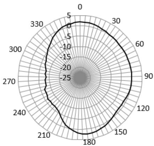
XY-2450MHz
