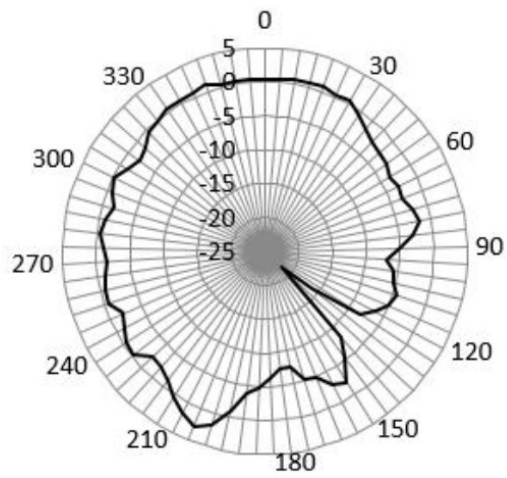
YZ-5450MHz
