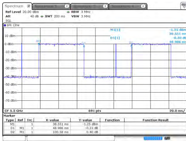
11a 5500 MHz
