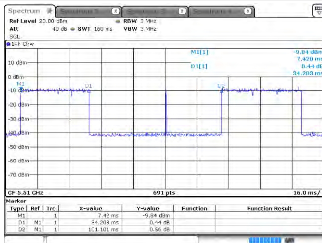
11n (HT40) 5510 MHz
