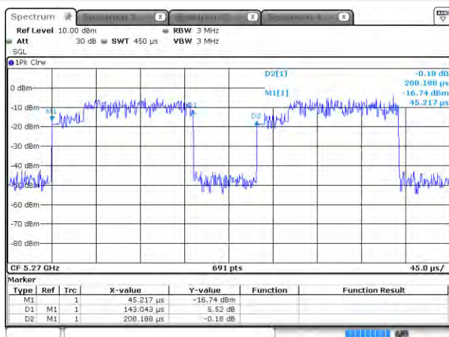
11n (HT40) 5270 MHz
