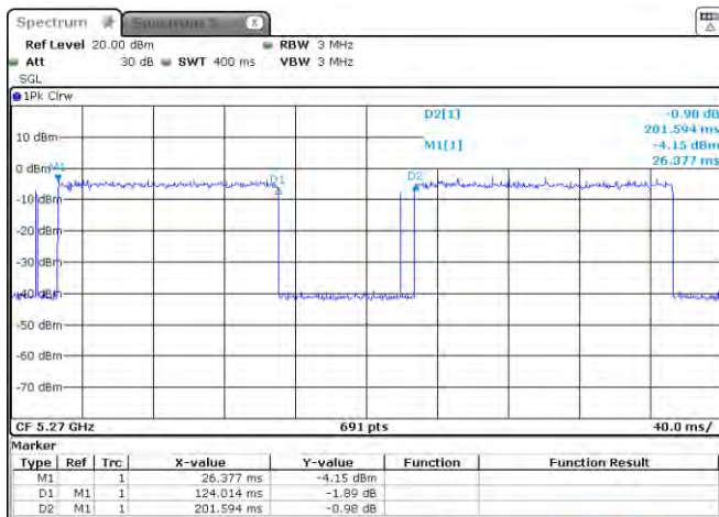
11n (HT40) 5270 MHz
