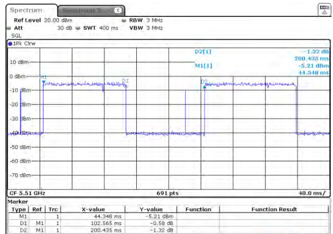
11n (HT40) 5510 MHz
