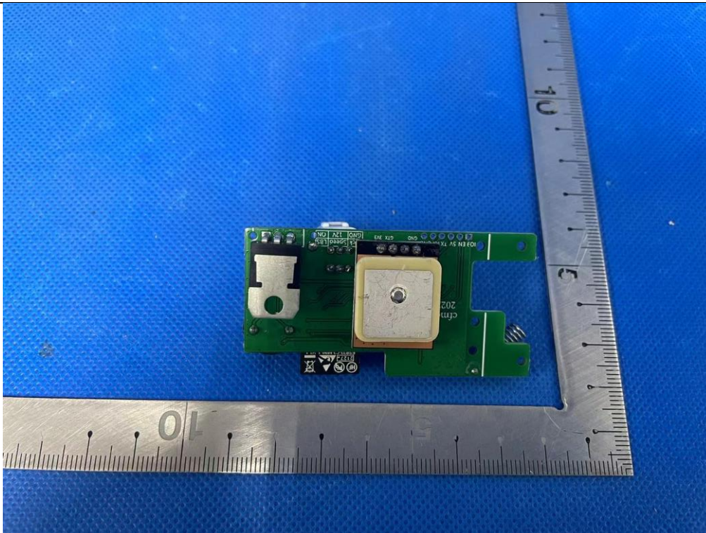
(2) EUT Photo(MCRMainControl)
