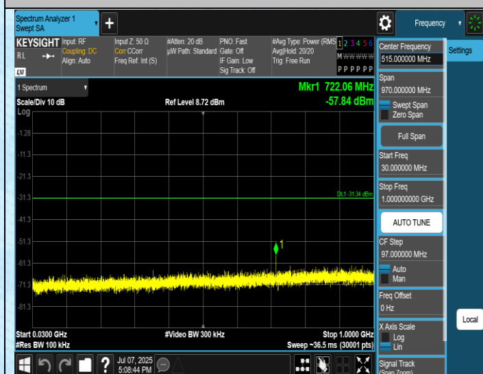
11N20MIMO-Ant4-2412-30~1000-PASS
