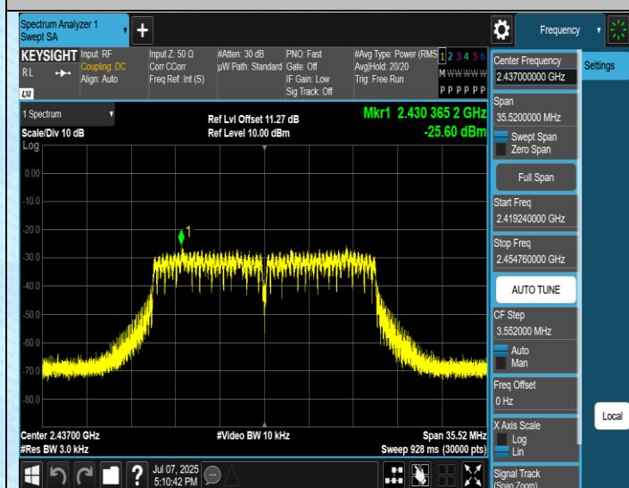
11N20MIMO-Ant3-2437-PASS
