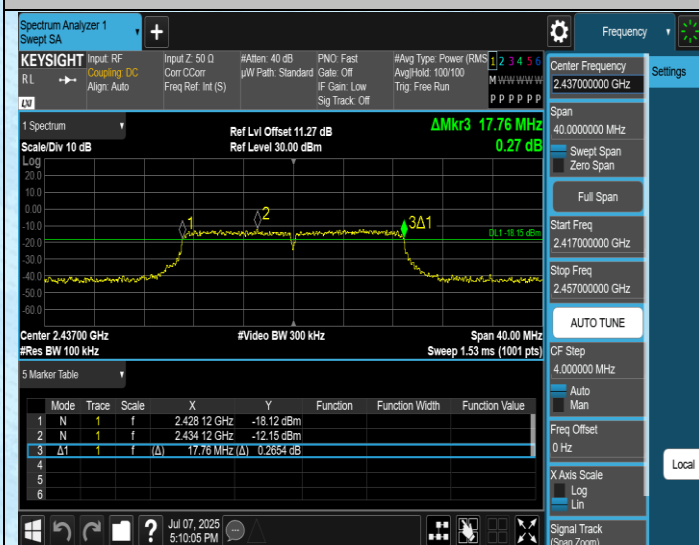
11N20MIMO-Ant3-2437-PASS
