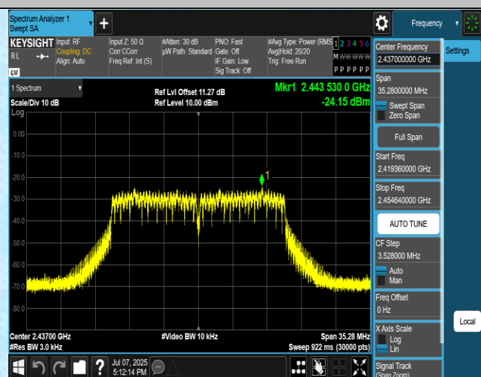
11N20MIMO-Ant4-2437-PASS
