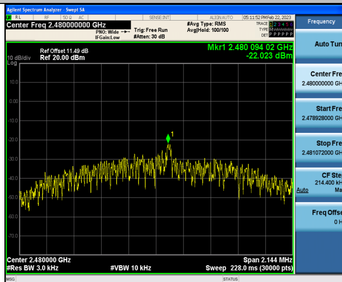
Mode2_2480
