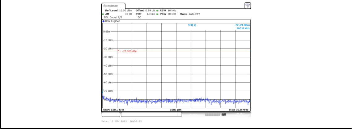
Band66-20MHz-QPSK-132572-1RB#0-Range2:0.15~30MHz
