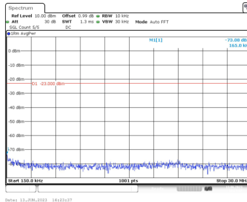
Band66-15MHz-QPSK-132597-1RB#0-Range2:0.15~30MHz
