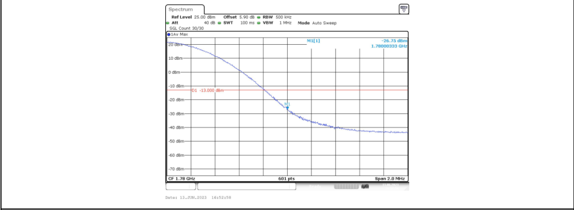
Band66-20MHz-QPSK-132572-1RB#99
