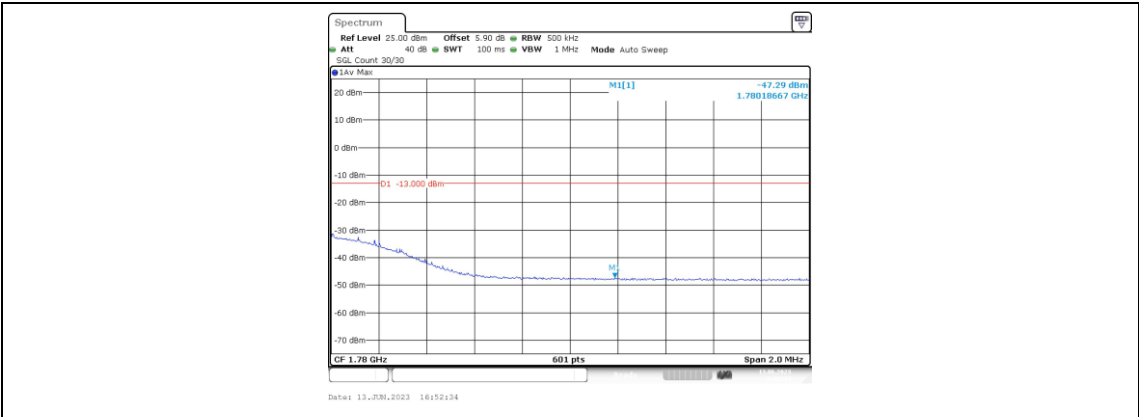
Band66-20MHz-QPSK-132572-1RB#0
