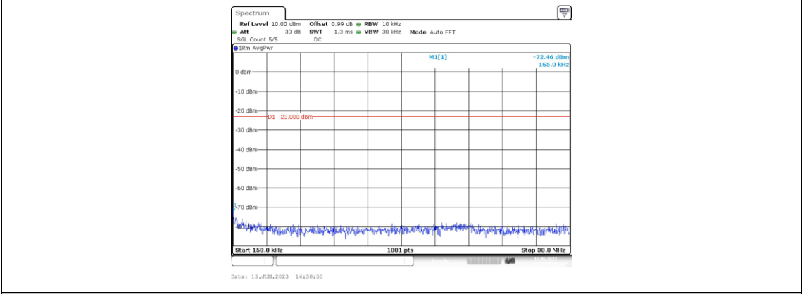
Band66-3MHz-QPSK-131987-1RB#0-Range2:0.15~30MHz
