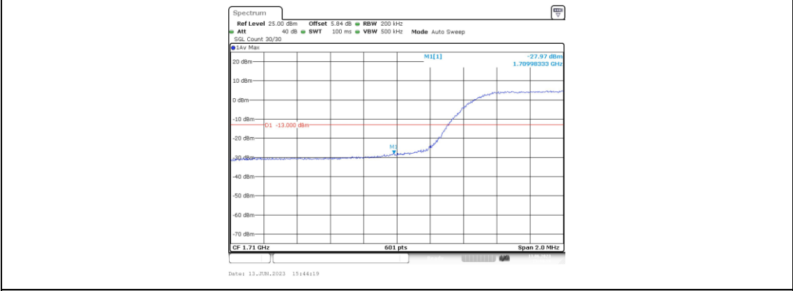
Band66-10MHz-QPSK-132022-50RB#0
