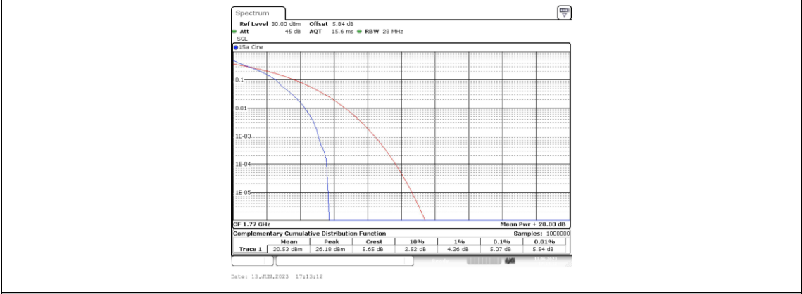
Band66-20MHz-QPSK-132572-1RB#0
