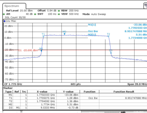
Band66-10MHz-QPSK-132622-50RB#0-8.952
