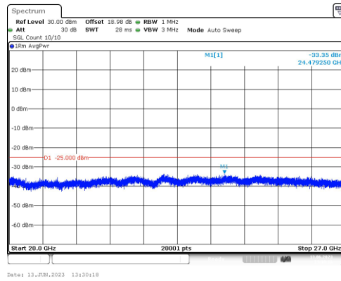
Band41-20MHz-QPSK-39750-1RB#0-Range5:20000~27000MHz
