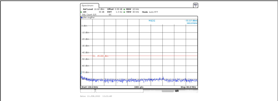
Band41-20MHz-QPSK-40620-1RB#0-Range2:0.15~30MHz
