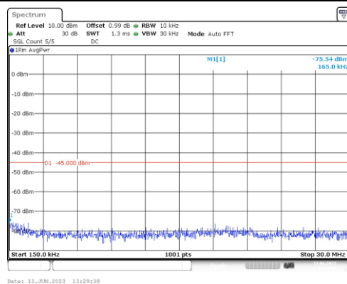
Band41-20MHz-QPSK-39750-1RB#0-Range2:0.15~30MHz
