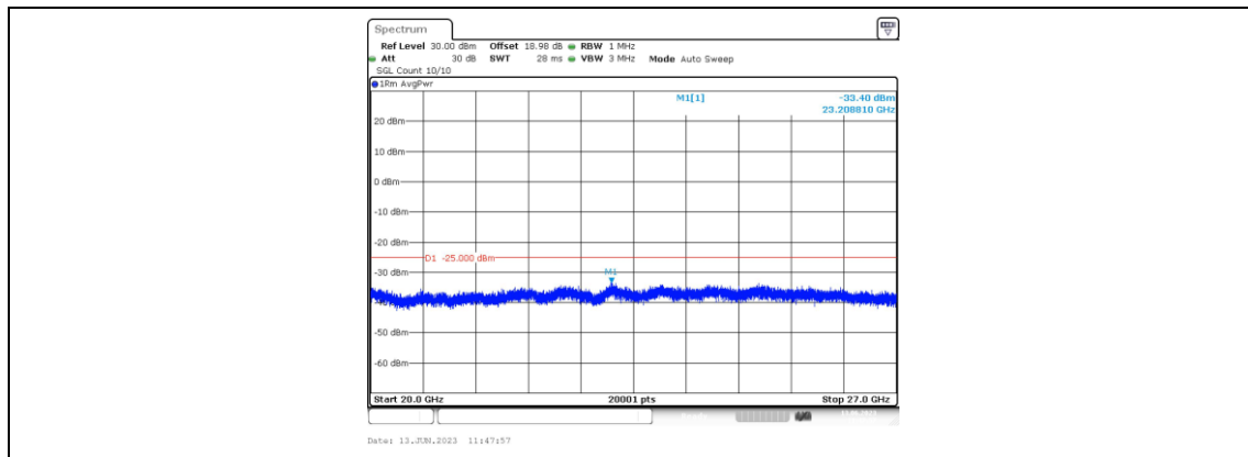
Band41-5MHz-QPSK-41565-1RB#0-Range5:20000~27000MHz
