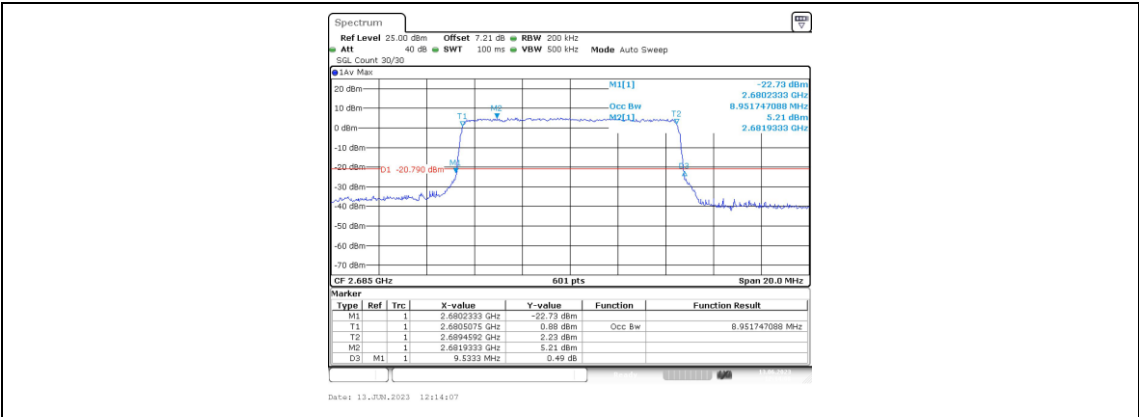
Band41-10MHz-QPSK-41540-50RB#0-8.952
