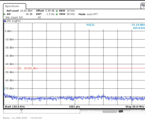
Band38-20MHz-QPSK-37850-1RB#0-Range2:0.15~30MHz
