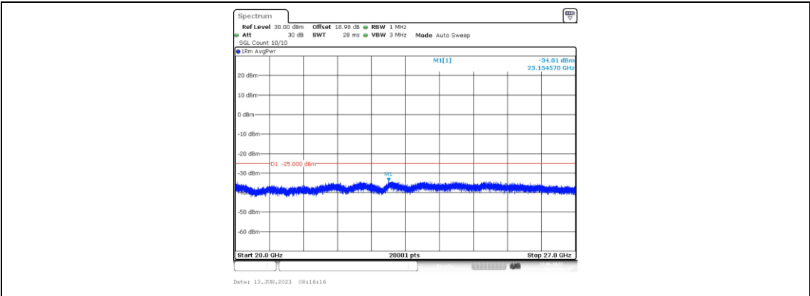
Band38-5MHz-QPSK-38225-1RB#0-Range5:20000~27000MHz
