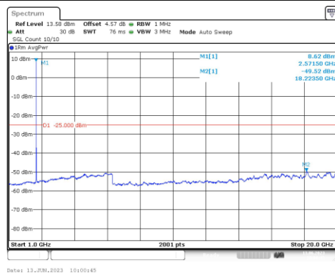
Band38-20MHz-QPSK-37850-1RB#0-Range4:1000~20000MHz
