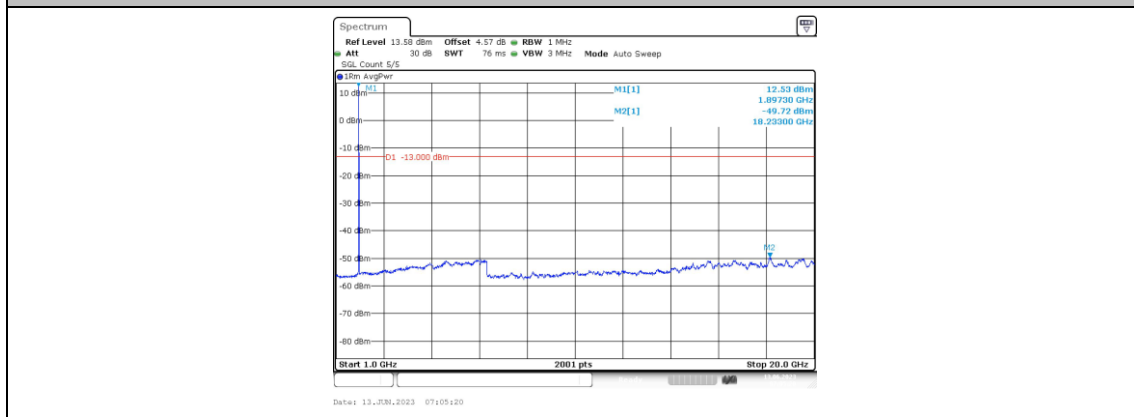
Band25-15MHz-QPSK-26615-1RB#0-Range4:1000~20000MHz
