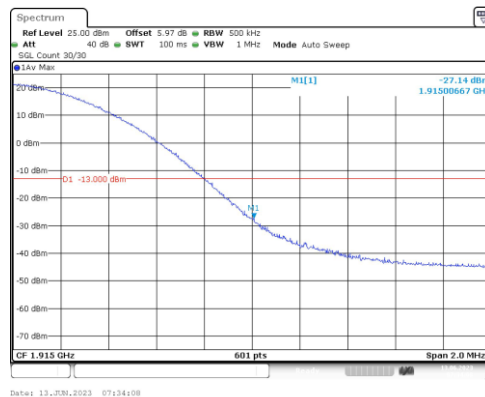
Band25-20MHz-QPSK-26590-1RB#99
