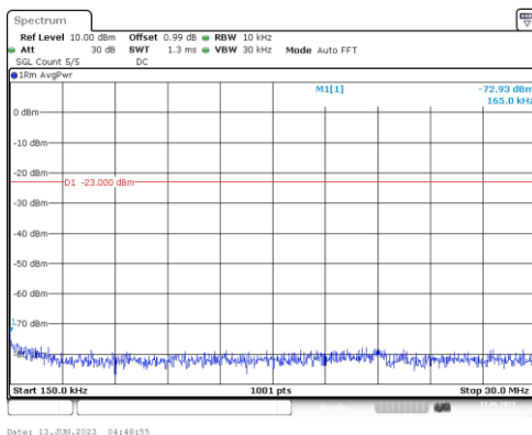
Band25-1.4MHz-QPSK-26047-1RB#0-Range2:0.15~30MHz
