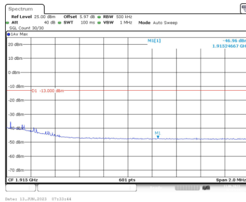
Band25-20MHz-16QAM-26590-1RB#0
