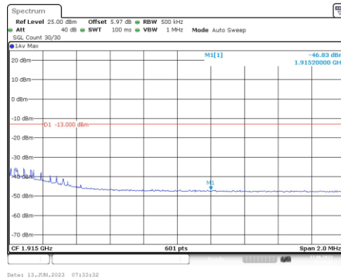
Band25-20MHz-QPSK-26590-1RB#0
