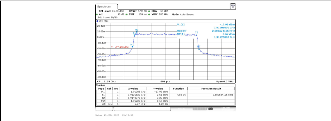
Band25-3MHz-QPSK-26675-15RB#0-2.686
