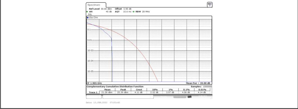
Band25-20MHz-QPSK-26590-1RB#0
