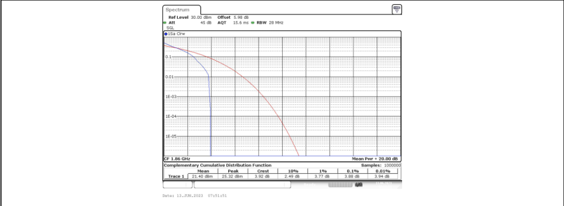
Band25-20MHz-QPSK-26140-1RB#0
