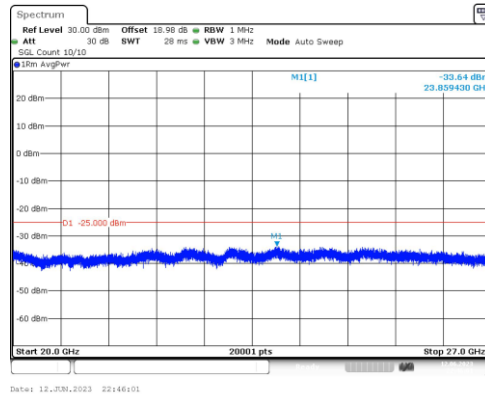
Band7-10MHz-QPSK-21400-1RB#0-Range5:20000~27000MHz
