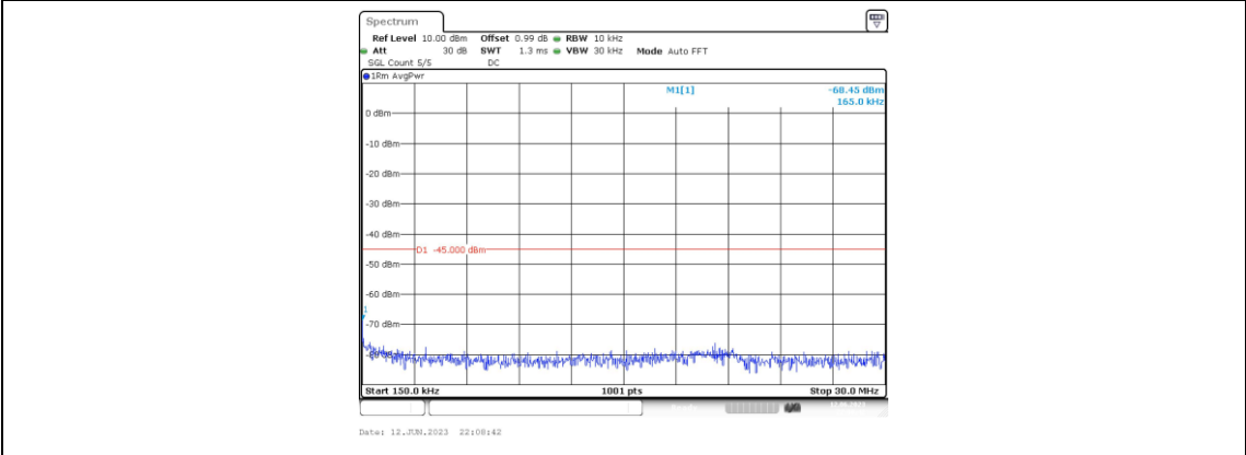
Band7-5MHz-QPSK-21100-1RB#0-Range2:0.15~30MHz
