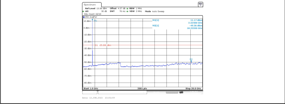
Band7-20MHz-QPSK-21100-1RB#0-Range4:1000~20000MHz
