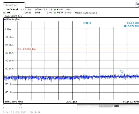
Band7-10MHz-QPSK-20800-1RB#0-Range3:30~1000MHz
