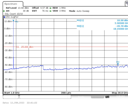
Band7-10MHz-QPSK-20800-1RB#0-Range4:1000~20000MHz
