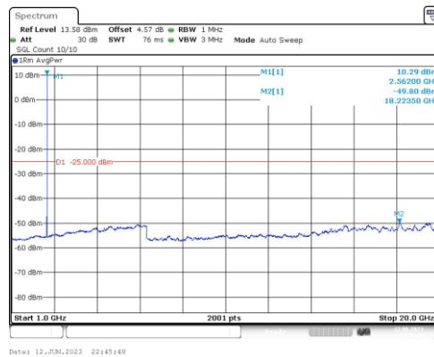
Band7-10MHz-QPSK-21400-1RB#0-Range4:1000~20000MHz
