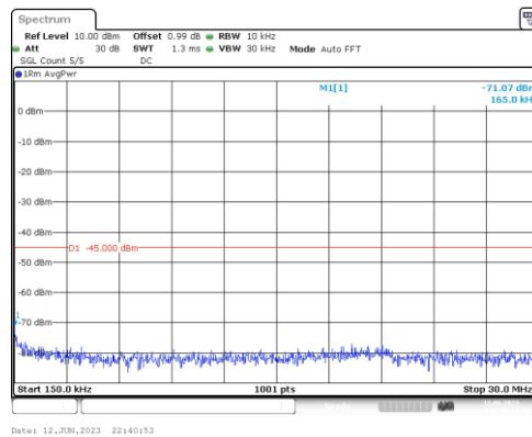
Band7-10MHz-QPSK-20800-1RB#0-Range2:0.15~30MHz
