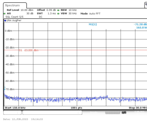
Band4-10MHz-QPSK-20175-1RB#0-Range2:0.15~30MHz
