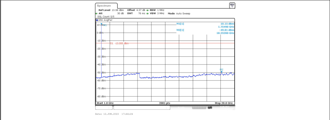
Band4-5MHz-QPSK-20375-1RB#0-Range4:1000~20000MHz
