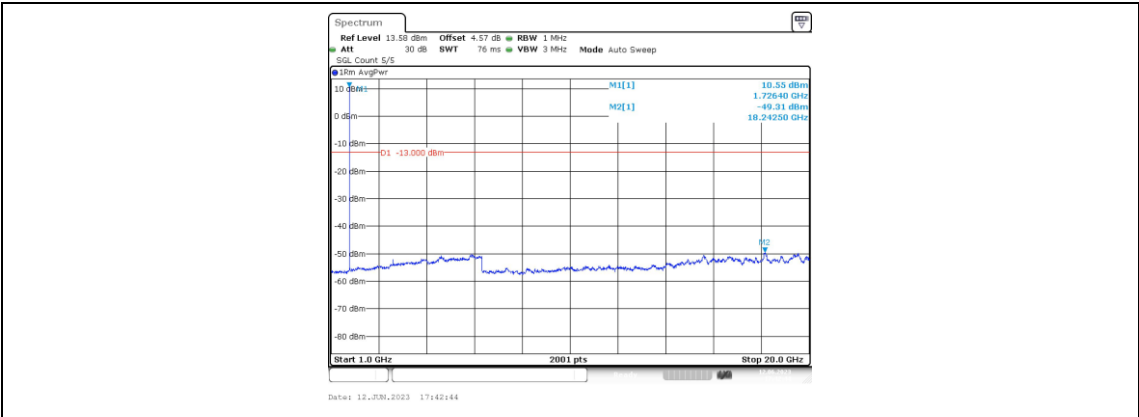
Band4-5MHz-QPSK-20175-1RB#0-Range4:1000~20000MHz
