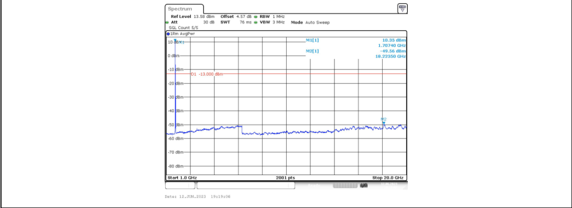
Band4-20MHz-QPSK-20050-1RB#0-Range4:1000~20000MHz
