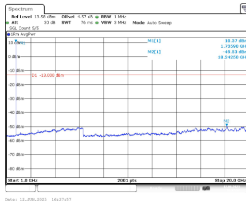
Band4-1.4MHz-QPSK-20175-1RB#0-Range4:1000~20000MHz
