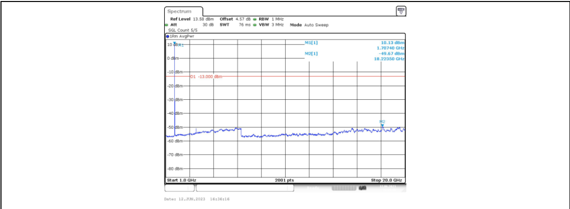
Band4-1.4MHz-QPSK-19957-1RB#0-Range4:1000~20000MHz
