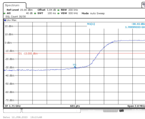
Band4-10MHz-QPSK-20000-50RB#0
