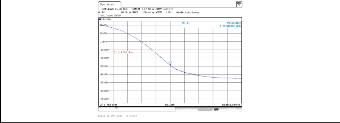
Band4-20MHz-QPSK-20300-1RB#99
