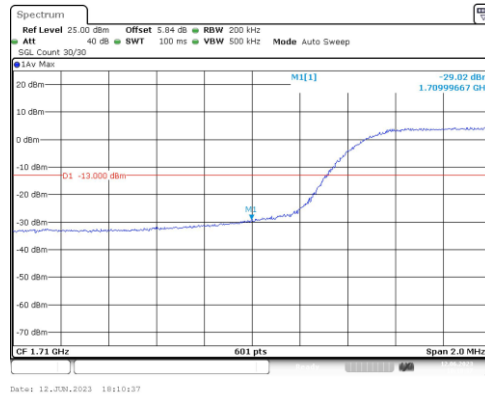
Band4-10MHz-QPSK-20000-50RB#0
