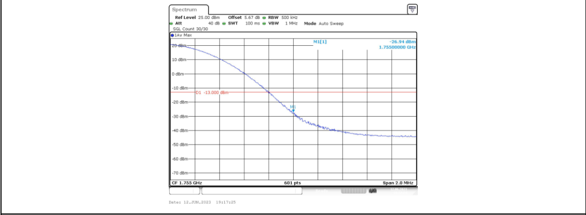
Band4-20MHz-QPSK-20300-1RB#99
