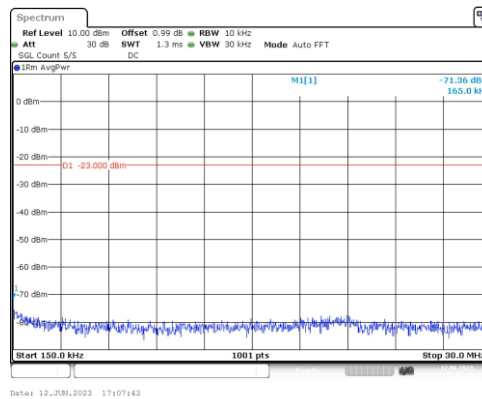
Band4-3MHz-QPSK-19965-1RB#0-Range2:0.15~30MHz
