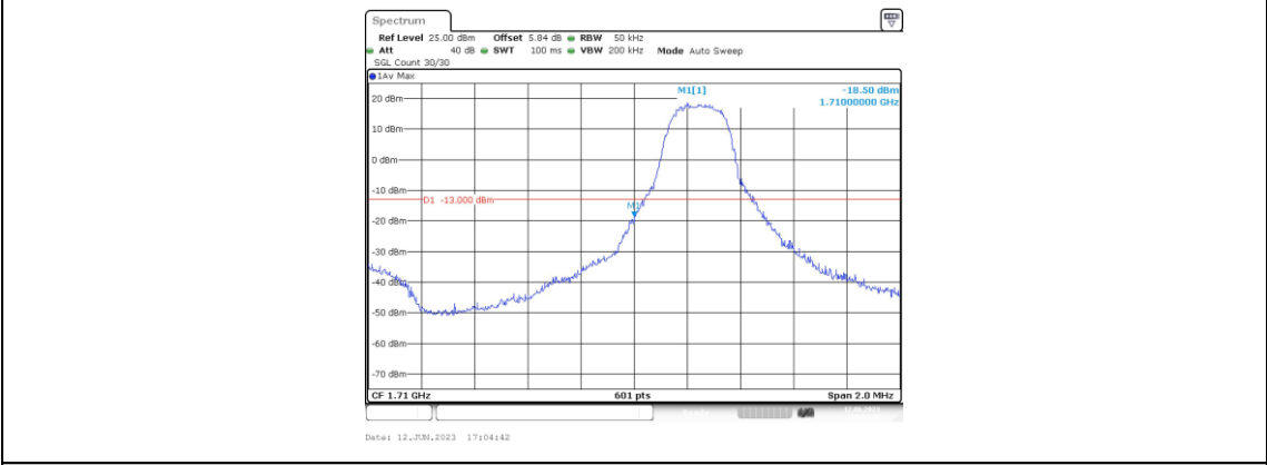
Band4-3MHz-QPSK-19965-1RB#0
