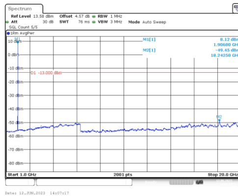
Band2-5MHz-QPSK-19175-1RB#0-Range4:1000~20000MHz
