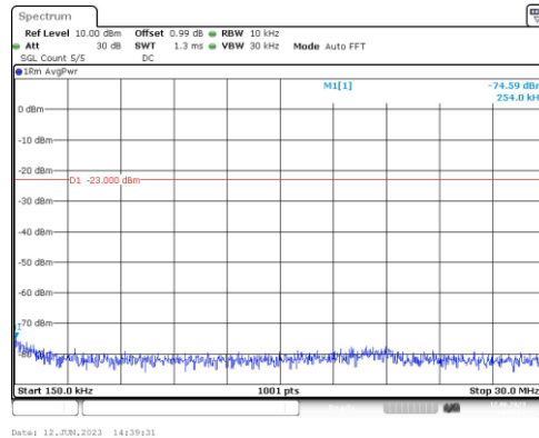
Band2-10MHz-QPSK-19150-1RB#0-Range2:0.15~30MHz
