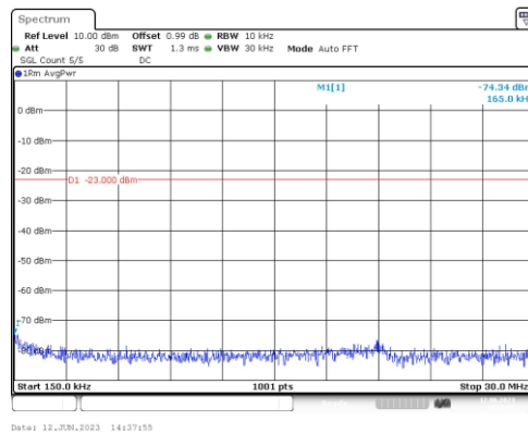
Band2-10MHz-QPSK-18900-1RB#0-Range2:0.15~30MHz
