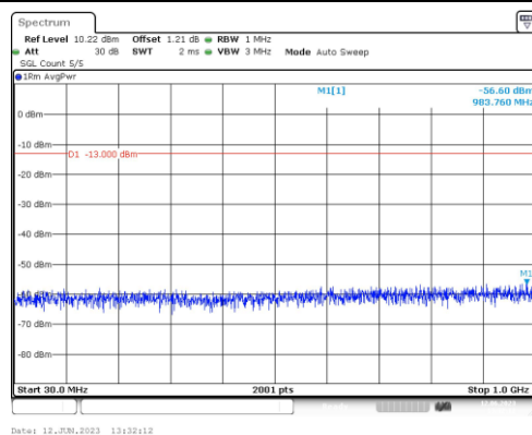
Band2-3MHz-QPSK-19185-1RB#0-Range3:30~1000MHz
