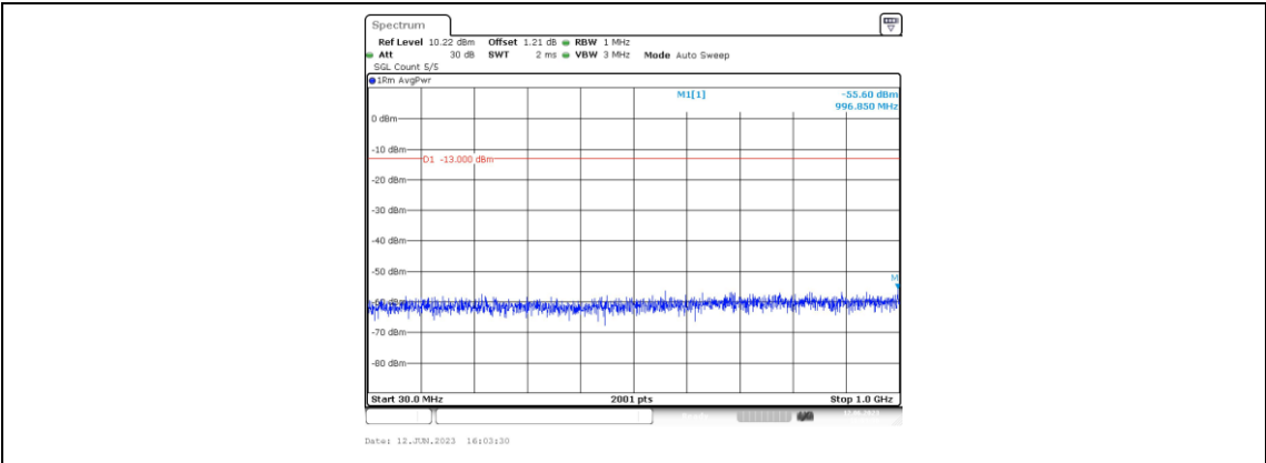
Band2-20MHz-QPSK-18700-1RB#0-Range3:30~1000MHz
