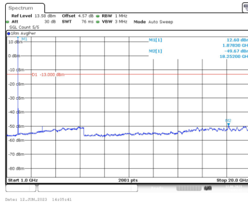
Band2-5MHz-QPSK-18900-1RB#0-Range4:1000~20000MHz
