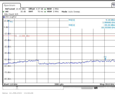
Band2-3MHz-QPSK-19185-1RB#0-Range4:1000~20000MHz
