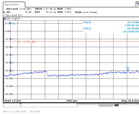
Band2-15MHz-QPSK-19125-1RB#0-Range4:1000~20000MHz
