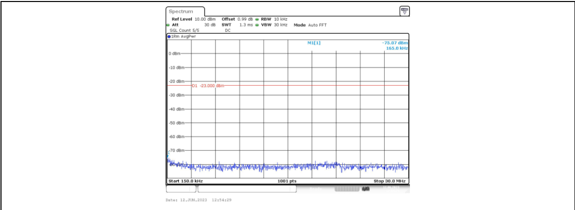
Band2-1.4MHz-QPSK-19193-1RB#0-Range2:0.15~30MHz
