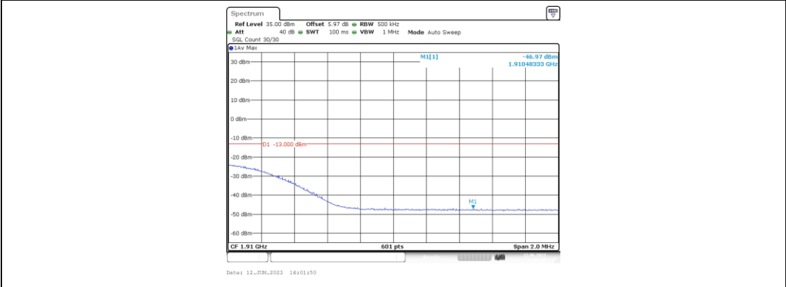
Band2-20MHz-16QAM-19100-1RB#0
