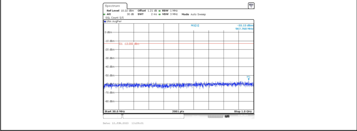
Band2-3MHz-QPSK-18615-1RB#0-Range3:30~1000MHz
