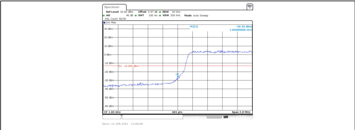
Band2-3MHz-16QAM-18615-15RB#0
