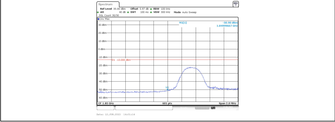
Band2-5MHz-QPSK-18625-1RB#24
