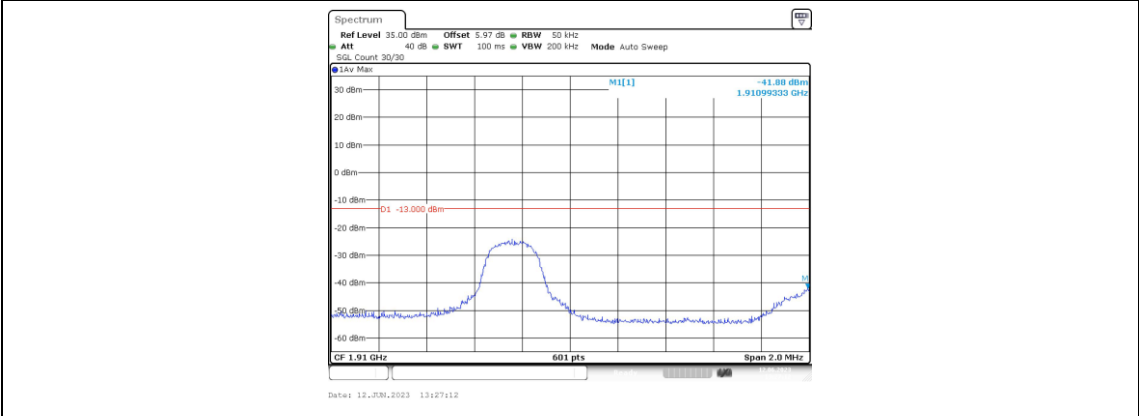
Band2-3MHz-QPSK-19185-1RB#0
