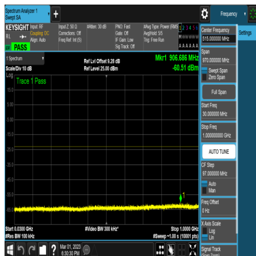
NTNV_N78-3450-3550_PC2_30_50_H_TID6_N/A _30_1000_#1
