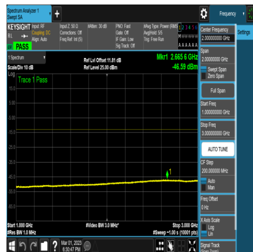
NTNV_N78-3450-3550_PC2_30_50_H_TID6_N/A _1000_3000_#1
