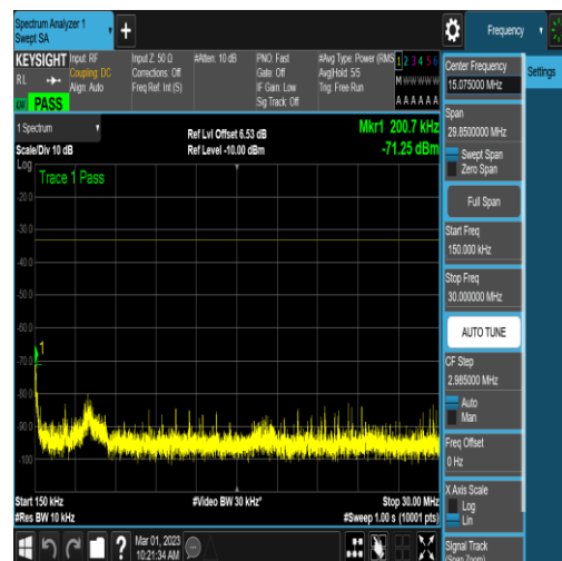
NTNV_N78-3450-3550_PC2_30_40_M_TID6_N/ A_0.15_30_#1
