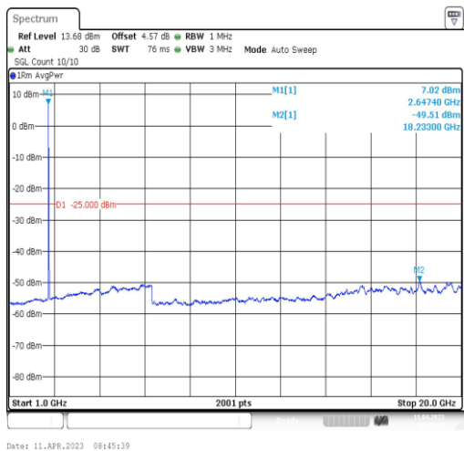
41-41-20MHz-20MHz-QPSK-QPSK-41292-41490-1RB#0-0RB#0-1000~20000MHz
