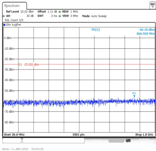
41-41-20MHz-20MHz-QPSK-QPSK-41292-41490-1RB#0-0RB#0-30~1000MHz
