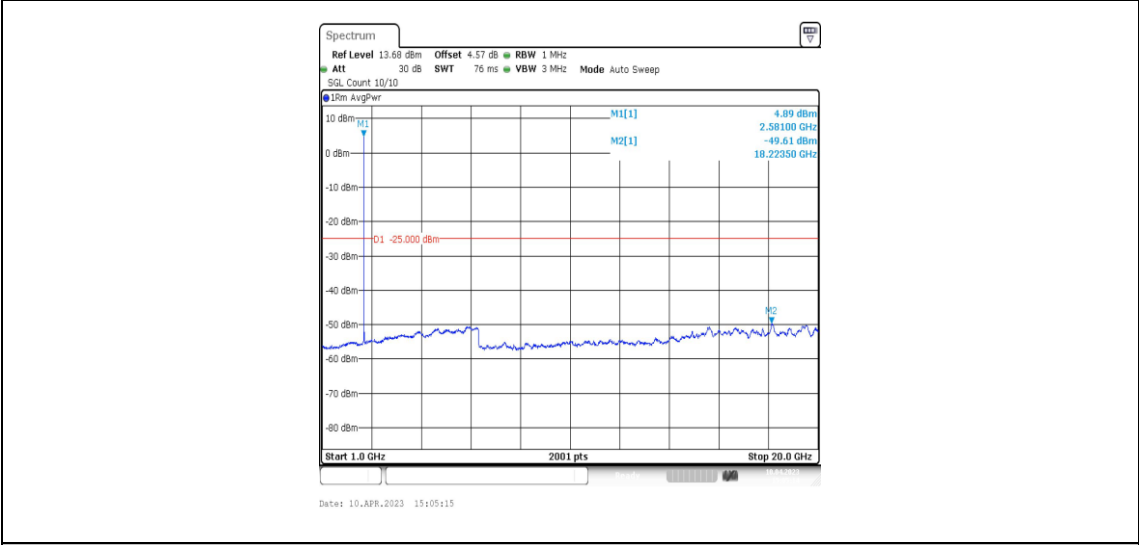
41-41-5MHz-20MHz-QPSK-QPSK-40528-40645-1RB#0-0RB#0-1000~20000MHz
