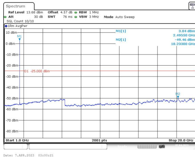
Band41-10MHz-QPSK-39700-1RB#0-Range5:20000~27000MHz
