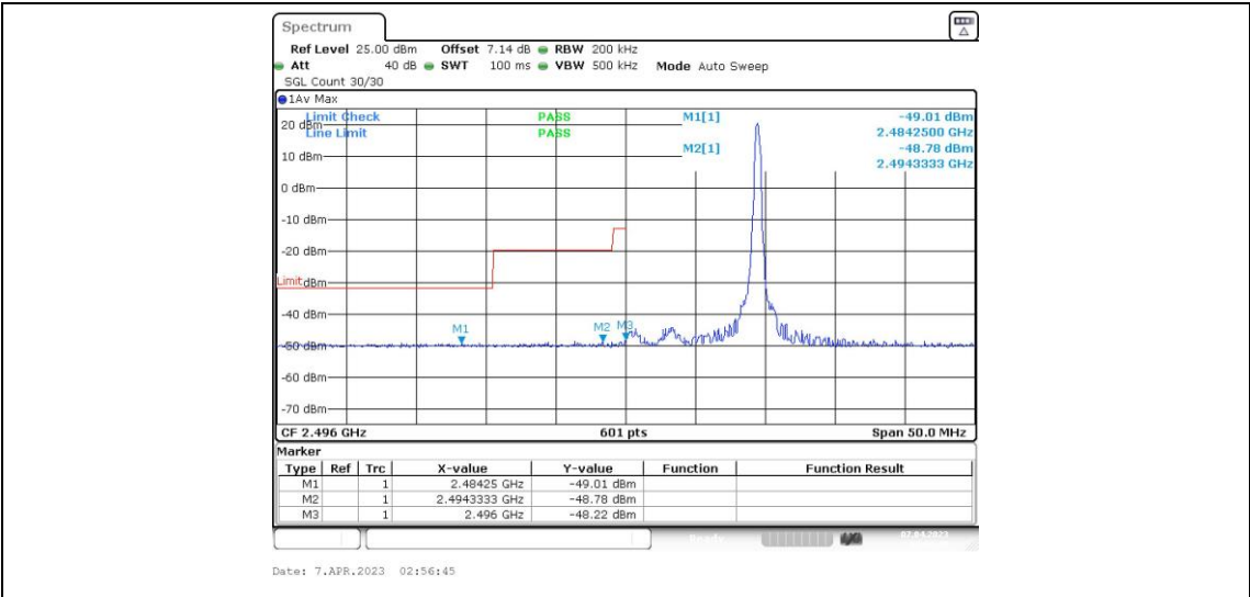
Band41-10MHz-QPSK-39700-50RB#0
