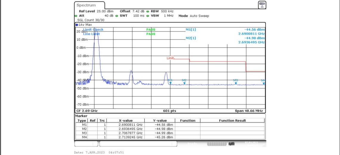
Band41-20MHz-QPSK-41490-1RB#99
