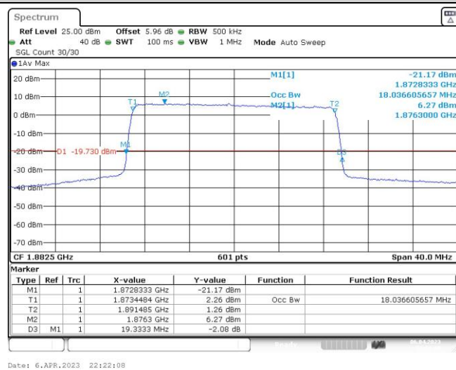
Band25-20MHz-QPSK-26590-100RB#0
