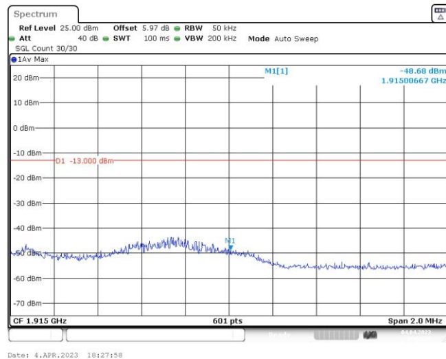
Band25-3MHz-QPSK-26675-1RB#14
