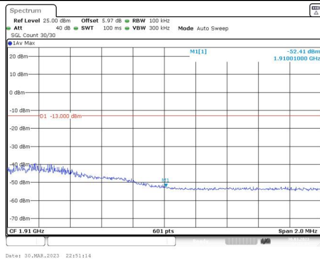
Band2-5MHz-QPSK-19175-1RB#24
