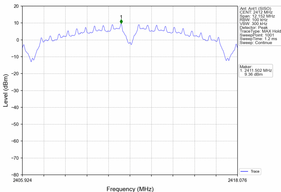
802.11b LCH 2412MHz Ant1 (SISO) NTN
