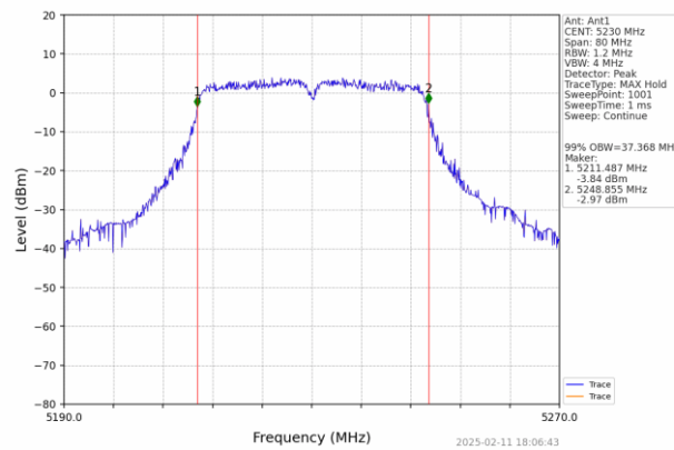
802.11n(HT40) HCH 5230MHz Ant1 NTN
