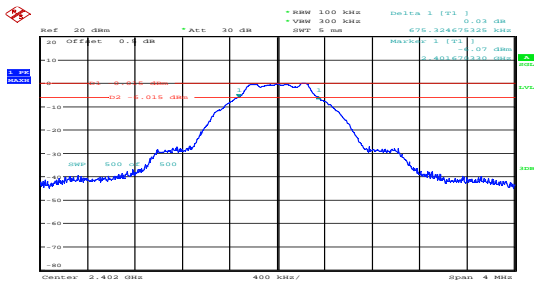
Low 0.675MHz
