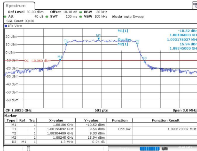
Band25-1.4MHz-QPSK-26365-6RB#0
