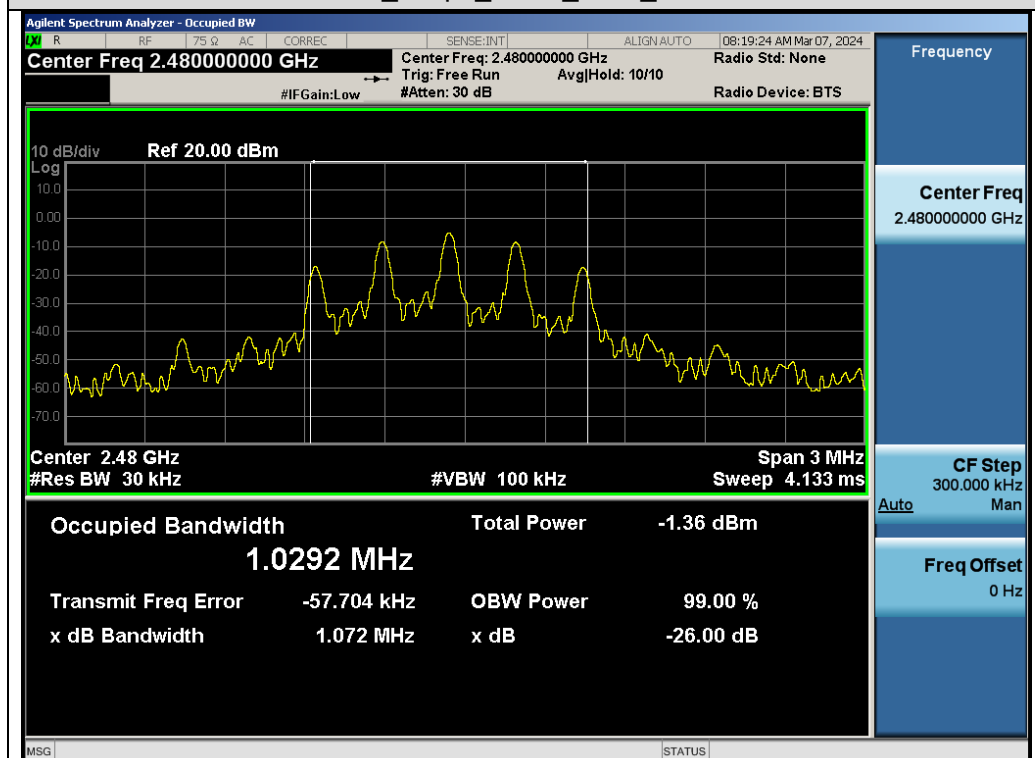
Test_Graph_ANT1_2480_OBW
