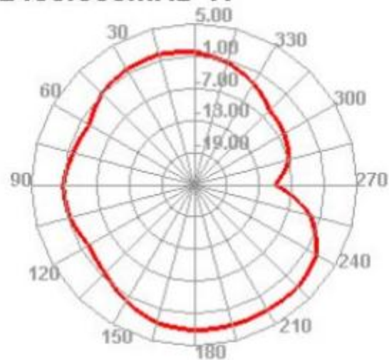
2450.000MHz H
