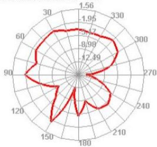
2450.000MHz H
