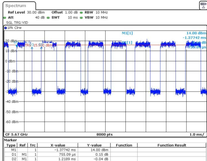
11AX40SISO_Ant1_5670
