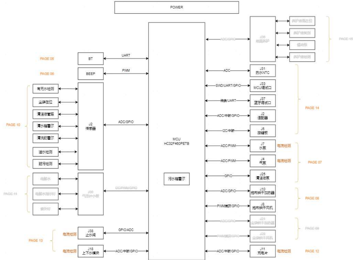
IP1207合芯方案基站主板框图 (基于1206修改)
